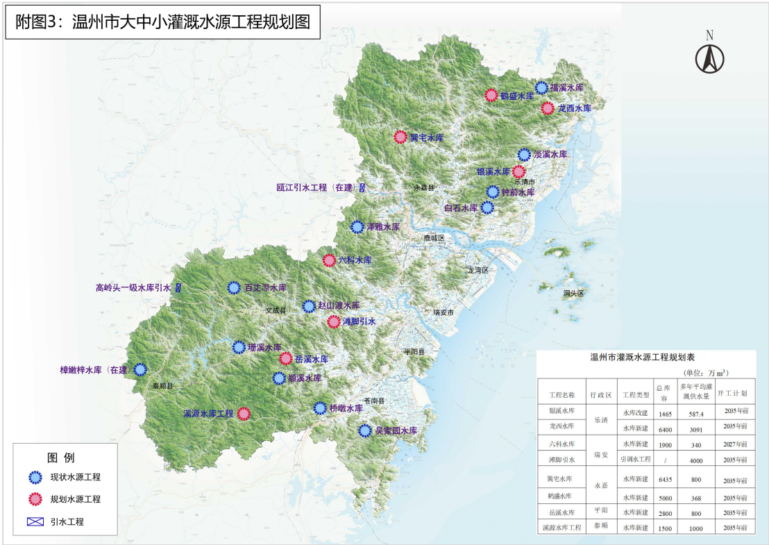
图 5.2-2 规划新建大中型水源工程布置图
