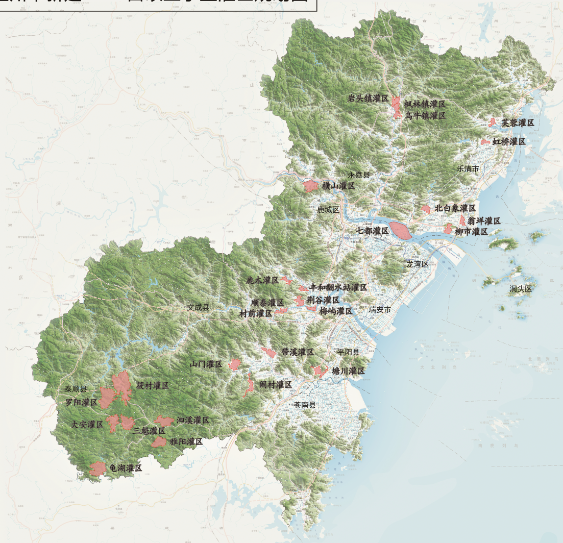
附图8 温州市新建2000亩以上小型灌区规划图
