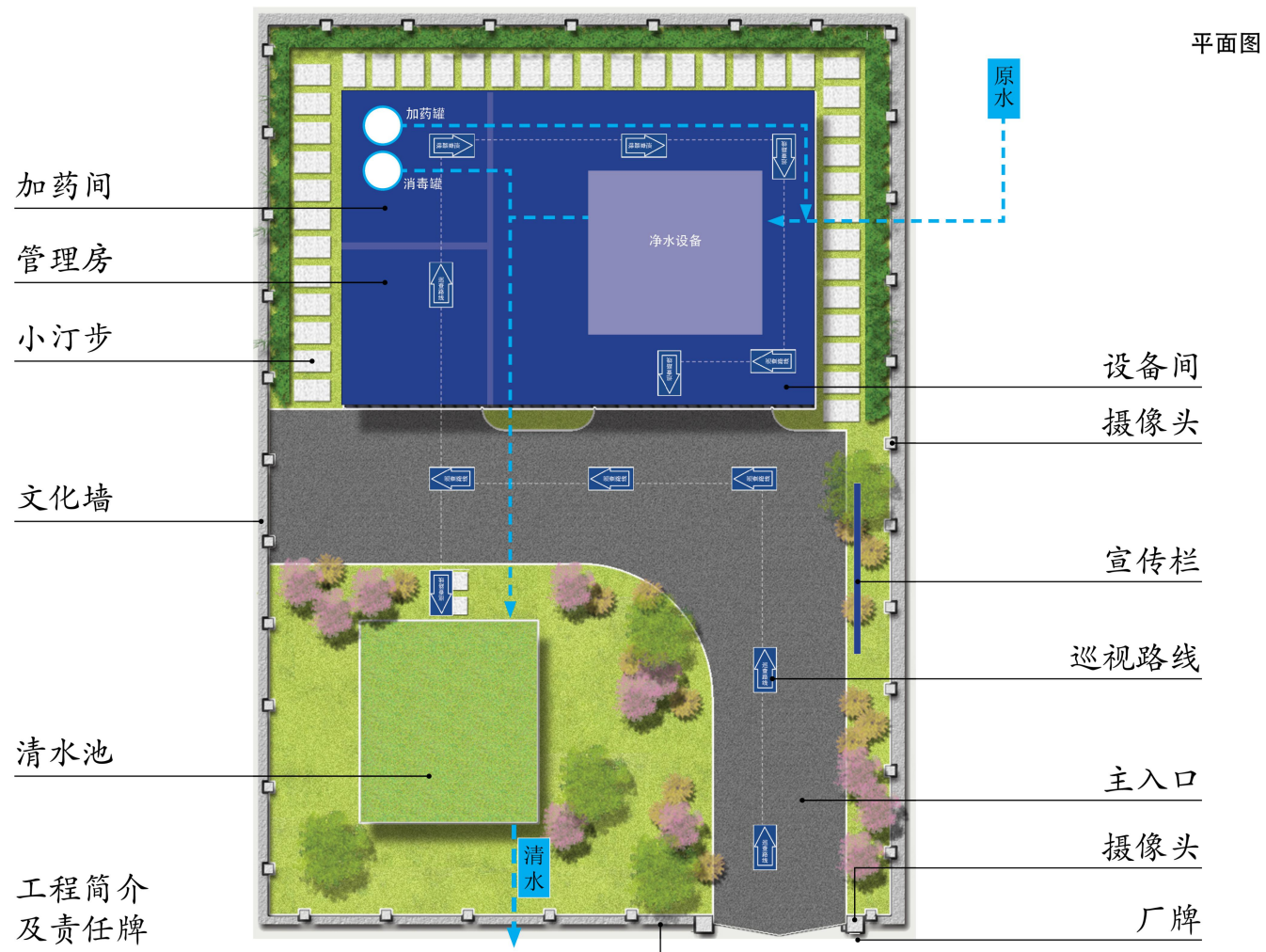
图 4 总平面图
